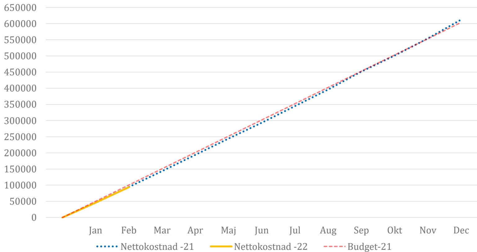
Nettokostnad
