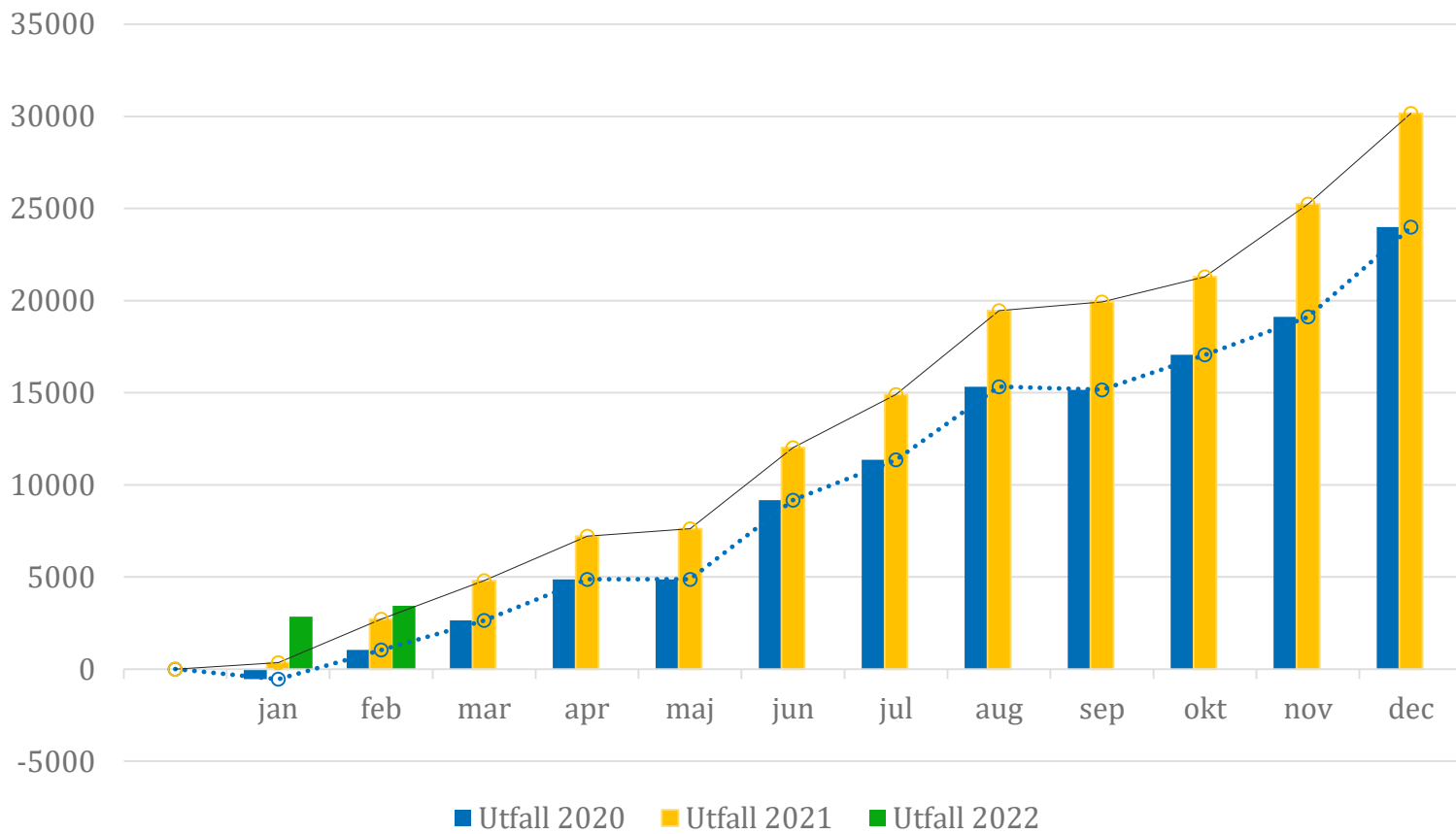
Diagramrubrik
