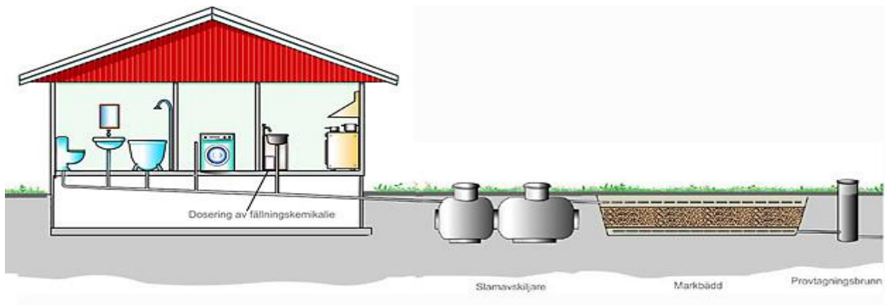
Bild: Principskiss för kemisk fällning i kombination med markbädd ( www.avloppsguiden.se )
