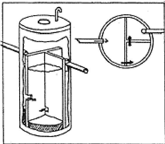
Bild: Slamavskiljare (genomskärning och från ovan)
